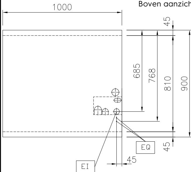
Boven aanzicht
